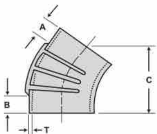
45° Elbow
