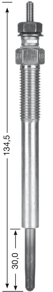
Y-527 J M 10 x 1.25 12 Hex 11 V DP 67
