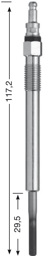
YE 14 M 8 x 1.0 8 Hex 4,4 V DP 48
