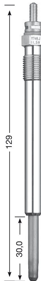
Y-746 J M 10 x 1.0 10 Hex 11,5 V DP 38
