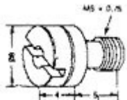
A-BAX Slot Jets
