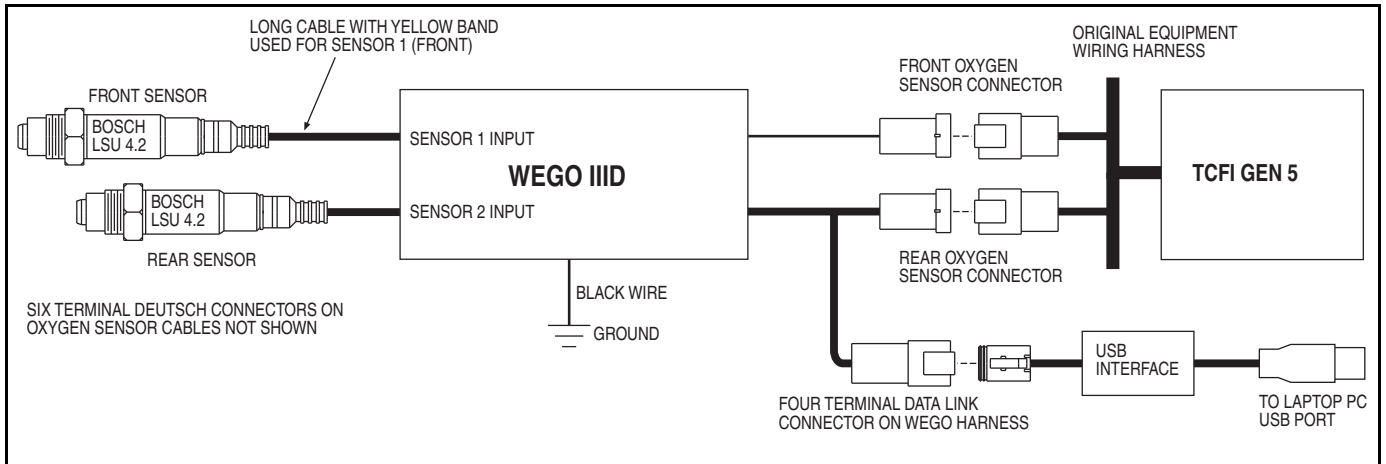
Figure 26 - WEGO Hookup
